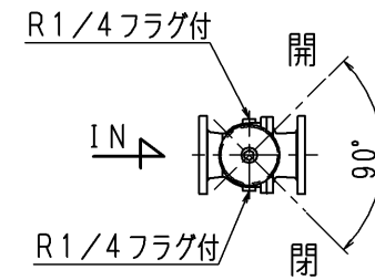
ボールコック開閉位置
